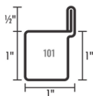
PERFIL TUBULAR 101 CALIBRE 20
